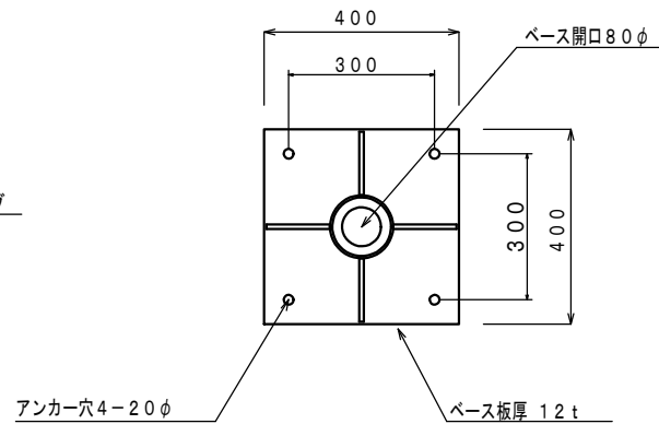
3. 5m~4mベースプレート詳細図
