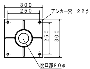
2m~3m ベース詳細図
